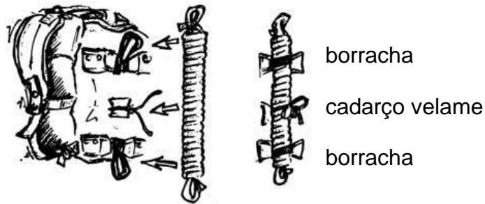
Fig 9 Acondicionamento do cabo solteiro
